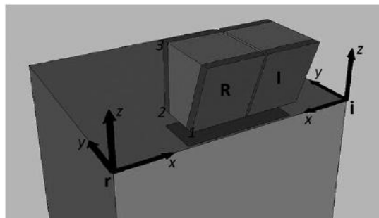
Figura 4. Ricostruzione tridimensionale del modello senza i mezzi di sintesi. R: colonna radiale, I: colonna intermedia. 1,2,3: punti di repere utilizzati per le misurazioni della colonna radiale (sono stati usati 3 punti di repere speculari per le misurazioni della colonna intermedia). r: centro di riferimento per le misurazioni della colonna radiale (x,y,z sono gli assi di riferimento). i: centro di riferimento per le misurazioni della colonna intermedia (x,y,z sono gli assi di riferimento).
