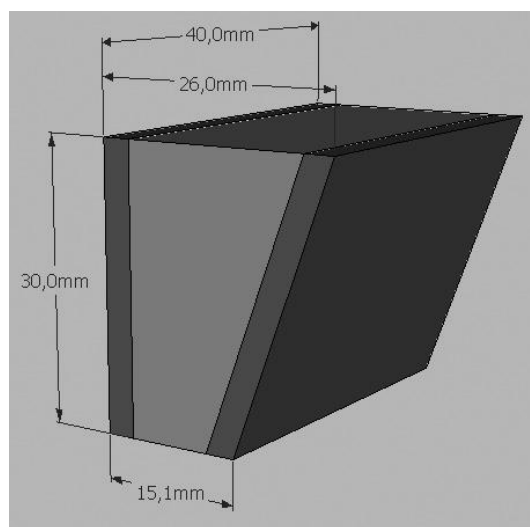
Figura 1. Ricostruzione tridimensionale del modello biomeccanico, con riportate le misure. E' composto da 2 strati esterni a maggior densità (50 pcf) e uno strato interno a minor densità (20 pcf).
