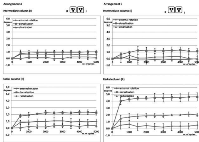
Figura 6. Scomposizione dei frammenti stabilizzati con la combinazione 4 e con la combinazione 5 (R: colonna radiale, I: colonna intermedia).
